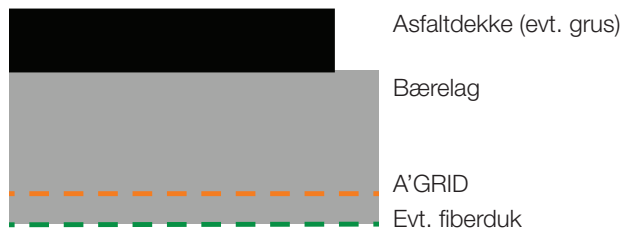
Figur 1. Typisk plassering av geonett i en veikonstruksjon ved forsterkning
